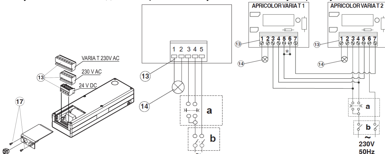
Рис.4. Электрическое подключение 220В
